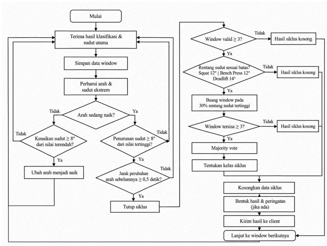
Gambar 3.5 Flowchart Modul Evaluasi Siklus Gerakan
