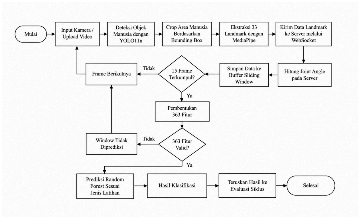
Gambar 3.3 Flowchart Modul Klasifikasi Postur
