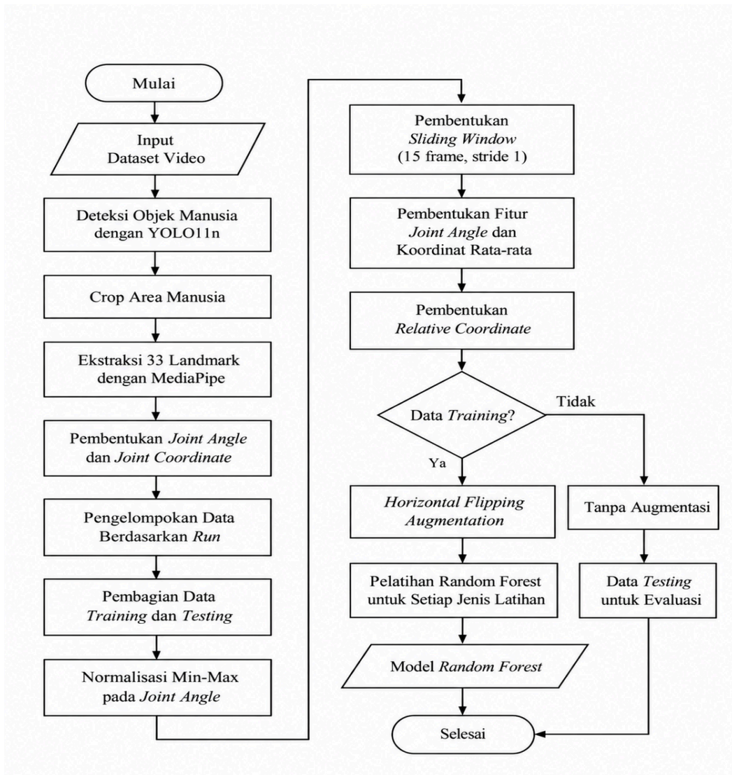
Gambar 3.2 Flowchart Modul Pengolahan Data dan Pelatihan Model
