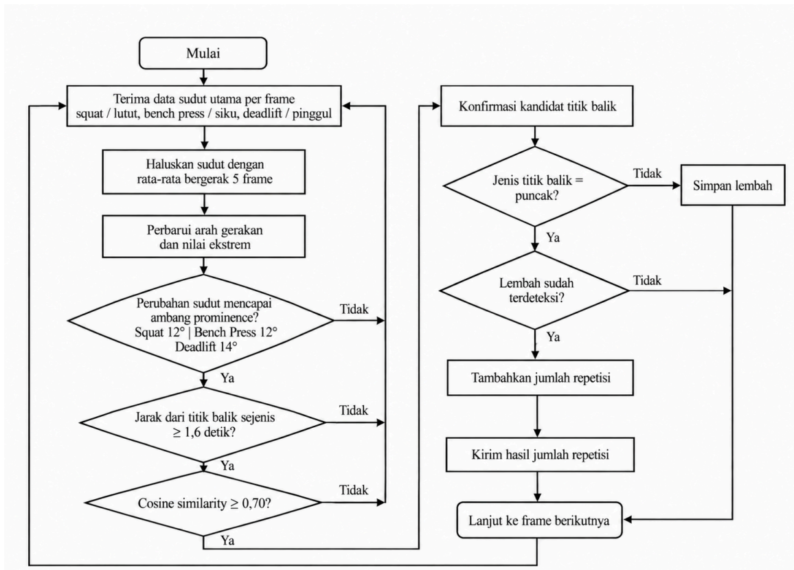
Gambar 3.4 Flowchart Modul Perhitungan Repetisi
